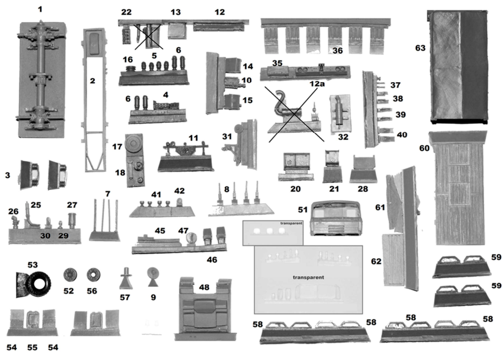
Tatra T815 4x4 VVN s plachtou
